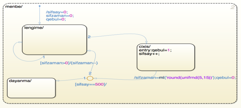
Şəkil 4. Mənbəbloğunun təsviri
