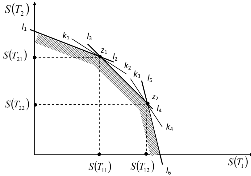
Şəkil 1.1. Xətti proqramlaşdırma məsələsinin qrafik təqdimatı.
