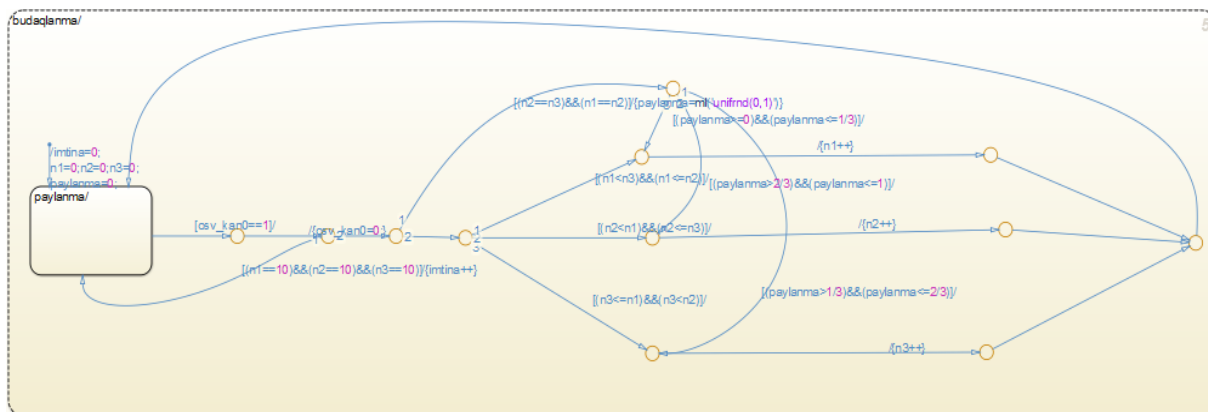
Şəkil 7. Sifarişlərin paylanma bloku
