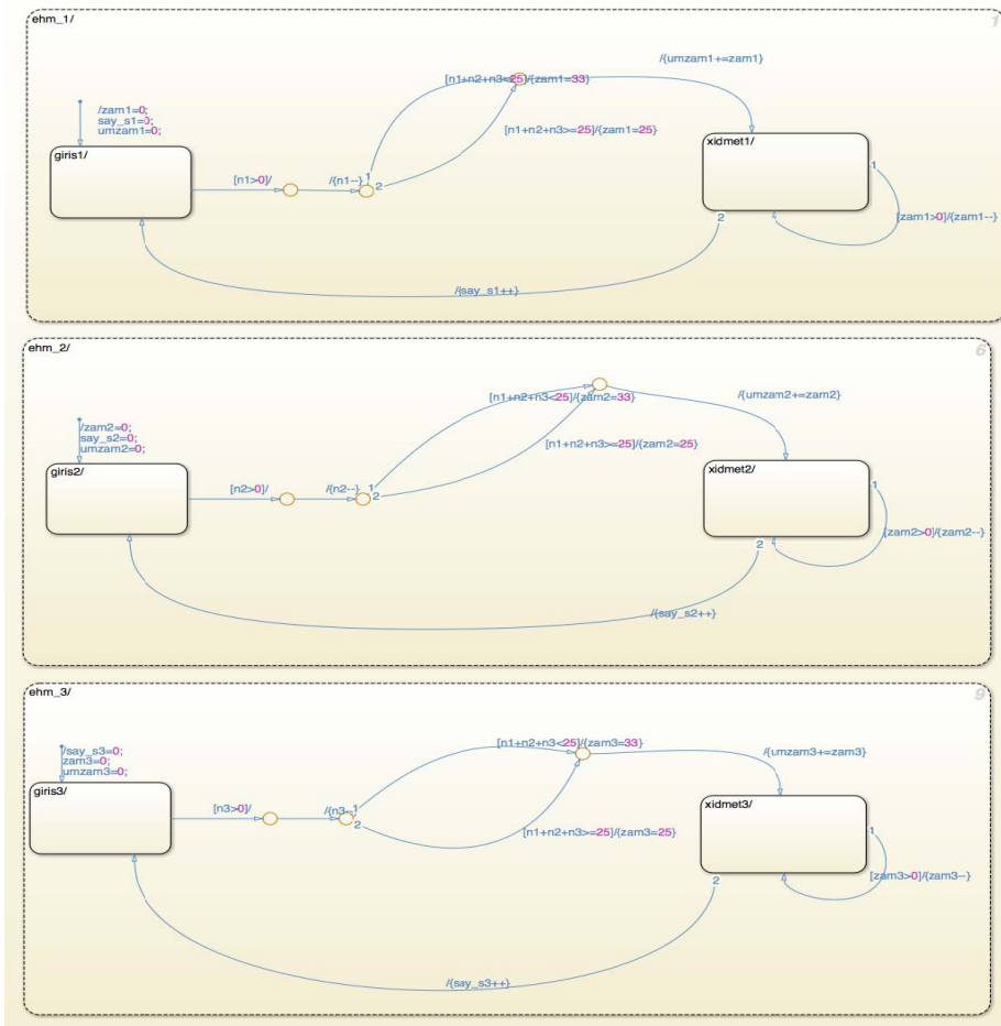
Şəkil 8. Mini EHM 1,2,3 blokları
