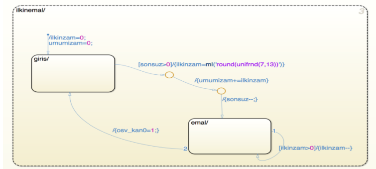
Şəkil 6. İlkin emal kanalı
