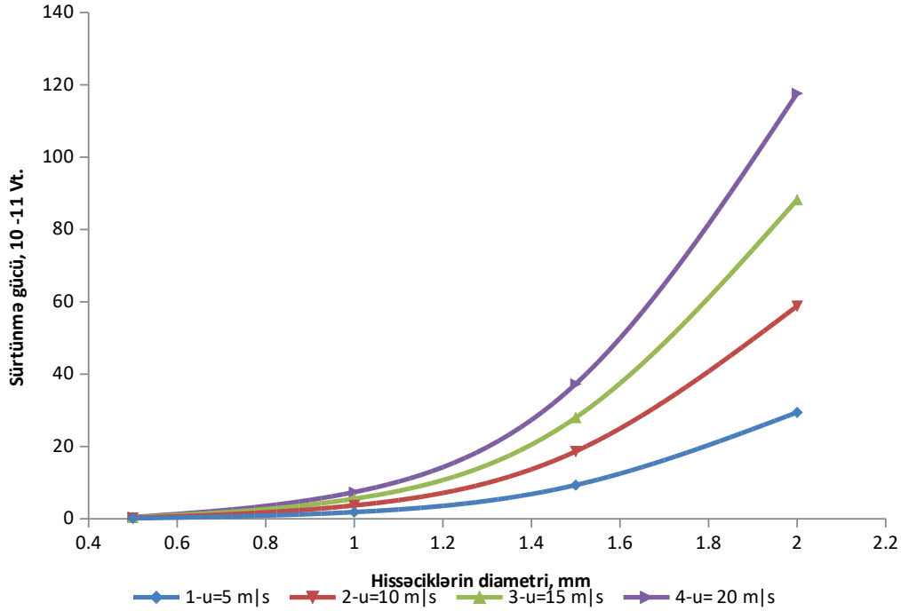
Şəkil 2. Mədən qaz-yığıcı xətlərində axının müxtəlif sürətlərində mexaniki hissəciklərdən yaranan sürtünmə gücünün hissəciklərin ölçüsündən asılılığı
