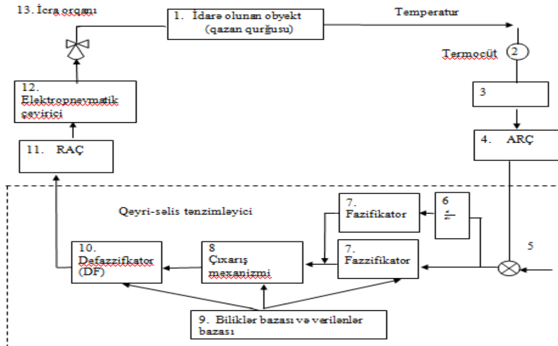
Şəkil 1. Qazan qurğusunun qeyri-səlis modelinin struktur sxemi
