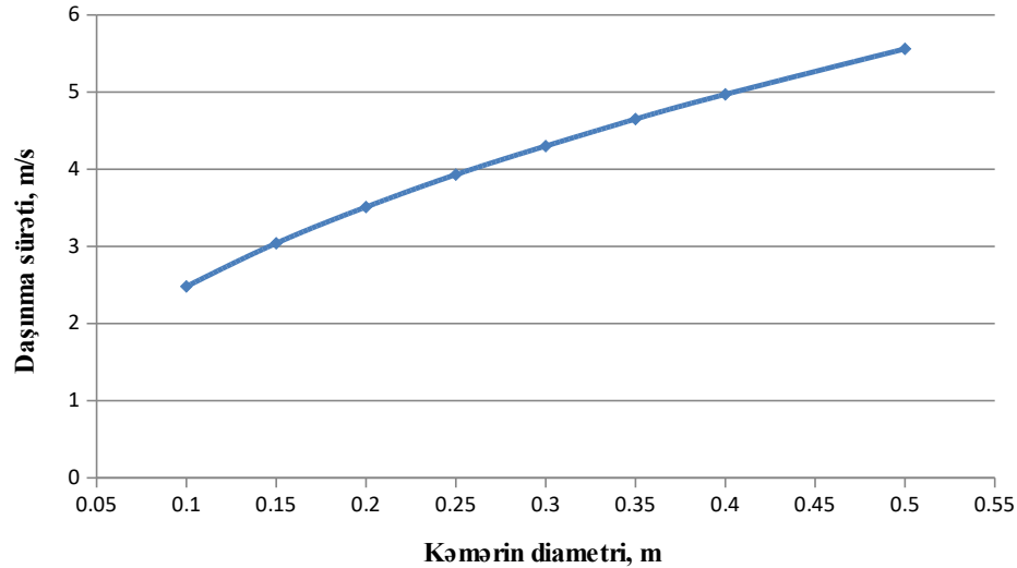
Şəkil 3. Qaz kəmərinə mexaniki hissəciklərin qaz axını ilə daşınma sürətinin kəmərin diametrindən asılılığı.
