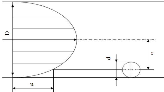
Şəkil 1. Mexaniki hissəciyin qaz axınında sürəti
