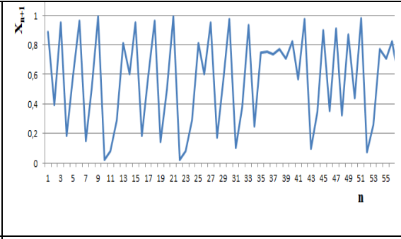
Şəkil 2, b. M_n psevdotəsadüfi ədədlər ardıcılığının qrafik təsviri ( r2=3.98 ; x_0=0.36 )
