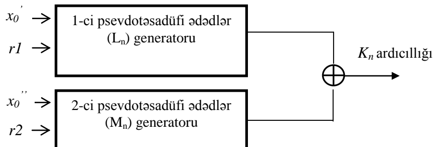
Şəkil 1. İki psevdotəsadüfi ədədlər ardıcılığı elementlərindən yeni psevdotəsadüfi ədədlər ardıcılığının alınmasının funksional sxemi
