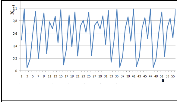
Şəkil 2, a. L_n psevdotəsadüfi ədədlər ardıcılığının qrafik təsviri ( r1=3.95 ; x_0=0.63 )
