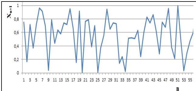
Şəkil 2, c. K_n psevdotəsadüfi ədədlər ardıcılığının qrafik təsviri
