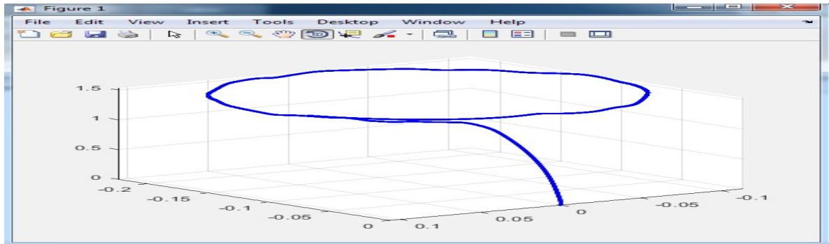
Şəkil 3.4. Kvadrotorun uçuş traektoriyası - x_{tap} = A \sin(\alpha t) , y_{tap} = A \cos(\alpha t) halı üçün
