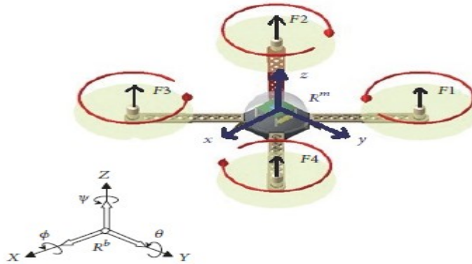
Şəkil 1.1. Kvadrotorun həndəsi modeli
