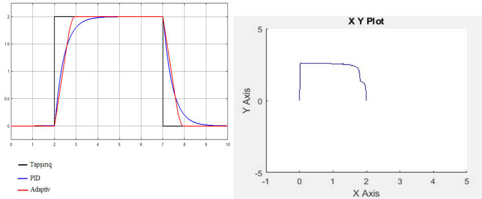
Şəkil 3.3. Kvadrotorun Eyer bucaqlarından birinin -\psi (yaw); x, y, z koordinatlarından birinin- y keçid prosesinin və onun faz portretinin qrafikləri
