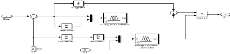
Şəkil 2.2. Qeyri-səlis adaptiv PDPİ tənzimləyicinin struktur sxemi
