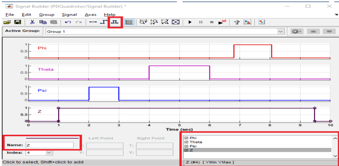
Şəkil 3.2. Kvadrotorun hərəkətinin-uçuşunun planlaşdırılmış trayektoriyasının zaman qrafikləri
