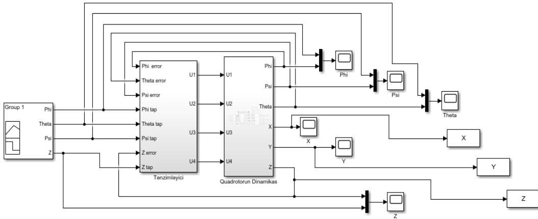
Şəkil 3.1. Kvadrotorun İİS-in MATLAB mühitində ümumiləşdirilmiş struktur sxemi
