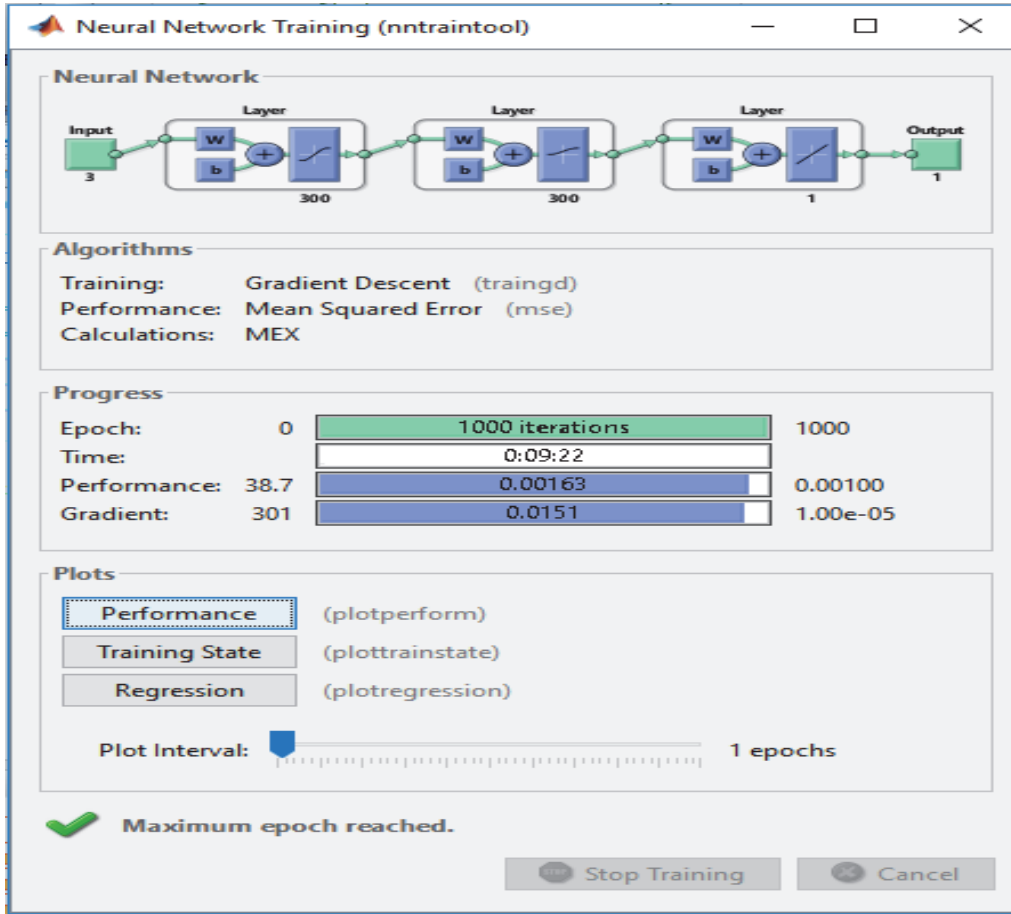
Şəkil 3.1. MATLAB mühitində “NNTtoolbox” da NŞ-in öyrədilməsinin (obyektin identifikasiyasının) parametrlərinin, informasiyaların təsviri
