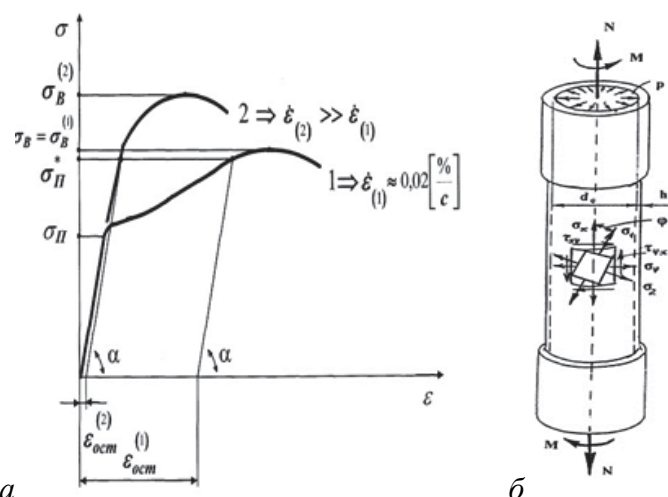
Рис.1. Комбинированное нагружение тонкостенного цилиндра
