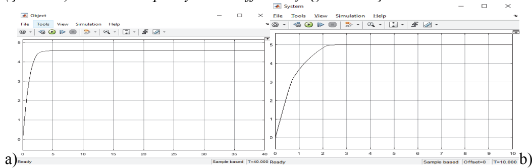
Şəkil 4.2. Real obyektin – mexatron qurğunun intellektual AİS-in (a) və NŞ tipli model əsasında intellektual AİS-in (b) keçid prosesləri
