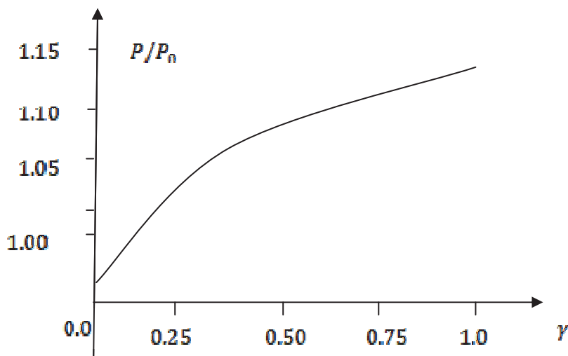
Şəkil 1. Böhran qüvvəsinin qeyri-bircinslik parametrindən asılılığı
