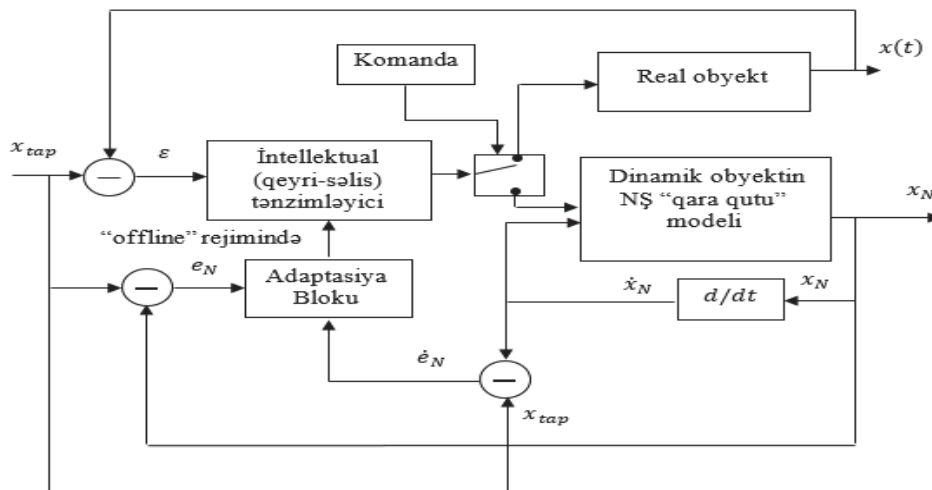
Şəkil 4.1. İntellektual qeyri-səlis tənzimləyicinin sazlama parametrlərinin (term çoxluqlarının modalarının) e_N və \dot{e}_N əsasında “offline” rejimdə adaptasiyasının strukturu
