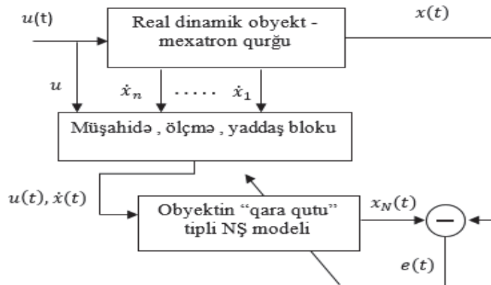
Şəkil 2.1. Vəziyyət dəyişənləri müşahidə olunan QMXX dinamik obyektin NŞ əsasında “qara qutu” şəklində modelləşdirilməsi sisteminin strukturu
