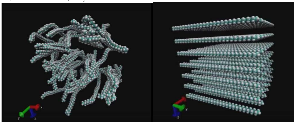
Şəkil 4. Gromacs-da əldə edilən molekulların qarşılıqlı təsirinin müxtəlif mərhələlərində polietilenin quruluşu
